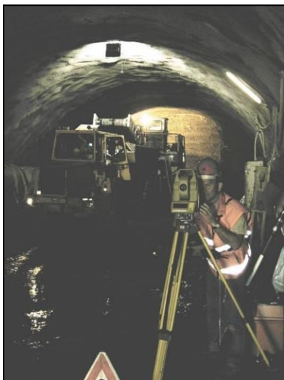
Messung Fixpunktnetz im Tunnel
