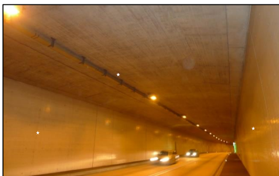
Konvergenzmessung im Tagbautunnel Ennetbaden
